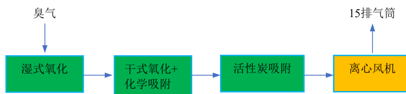
图 6.1-1 项目废气处理措施示意图
