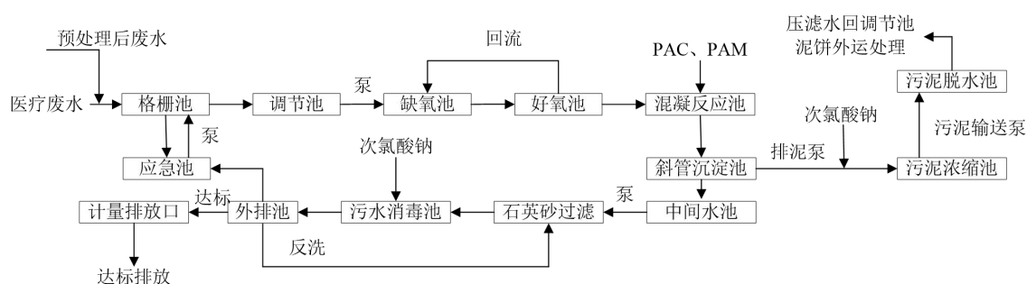
图 6.2-1 污水处理站工艺流程图
