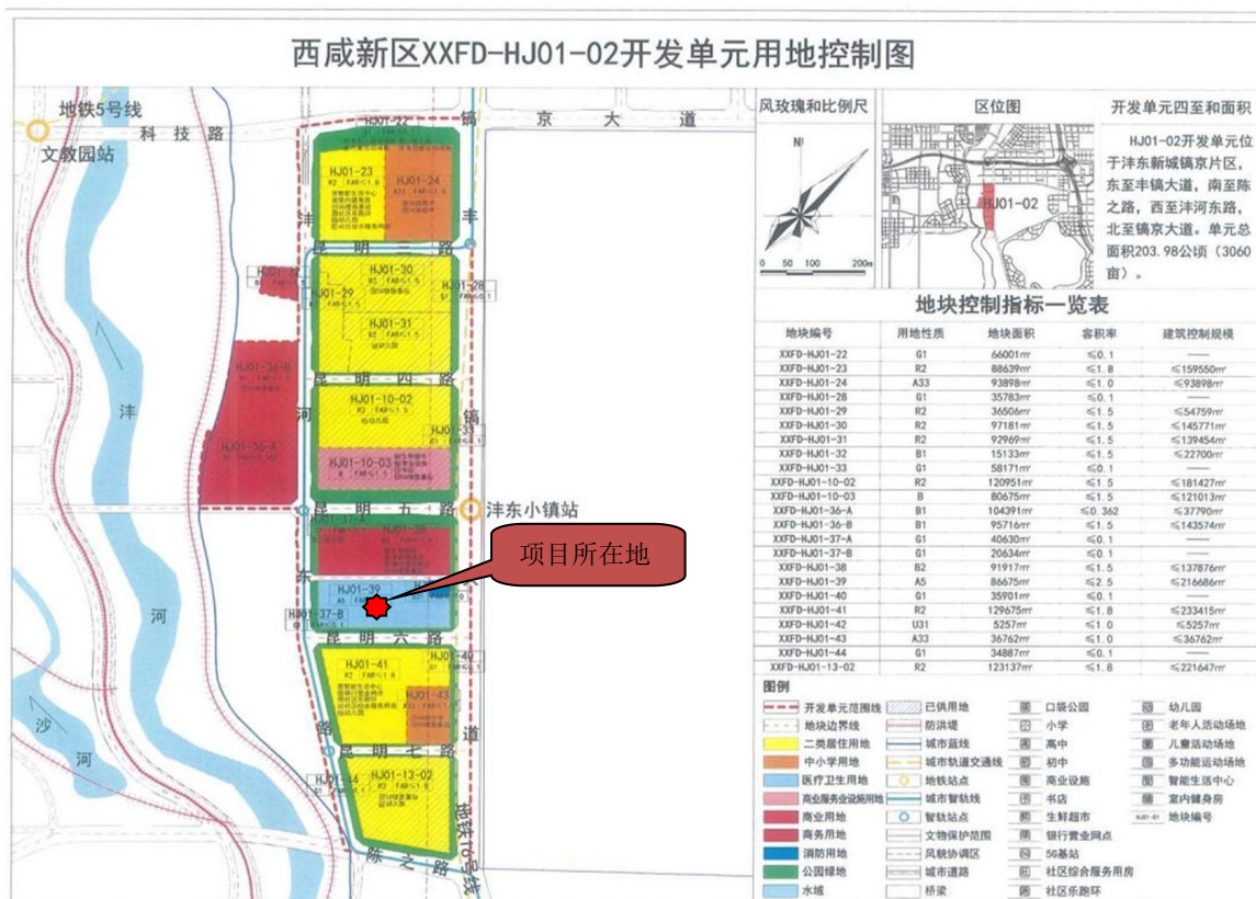
图 1.4-1 土地利用规划图
