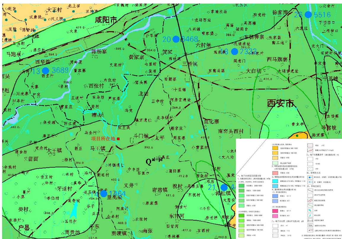
图 4.1-2 区域水文地质图
