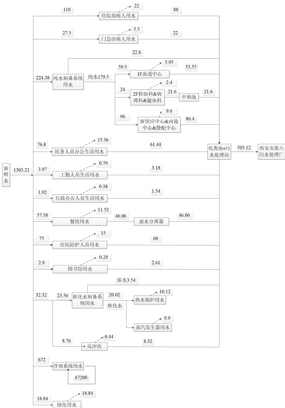
图 3.1-1 本项目水平衡图单位：m³/d
